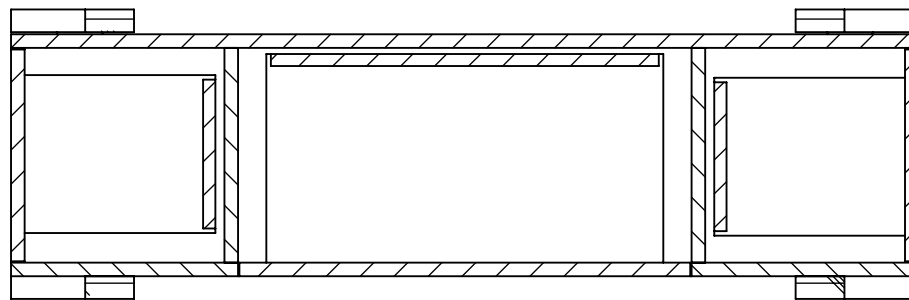
SECTION D-D SCALE 1 : 10
